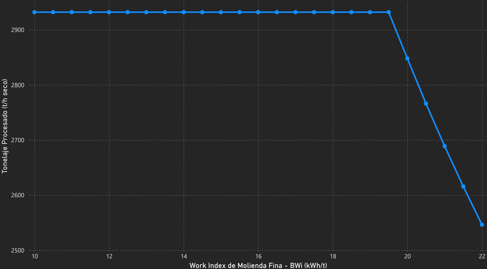
Análisis de Sensibilidad de Conminución: BWi vs. Capacidad Nominal
